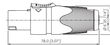
NA4LJX
