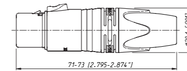
NC10MXX-14-B
