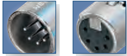
5芯公头连接器 5芯母头连接器
