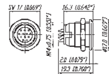
MPF(M)12-H
