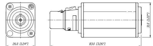
NADITBNC-FX
