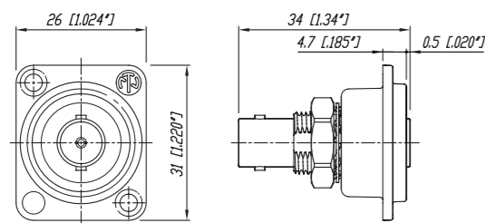
NBB75DFGX
