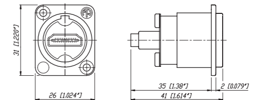
NAHDMI-W
