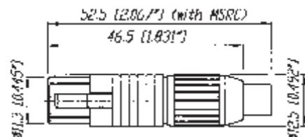
MSCF(M)12 (+MSRC)
