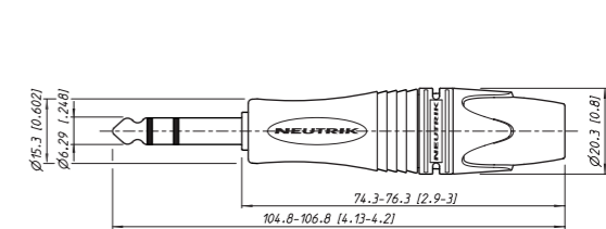
NP3XL
