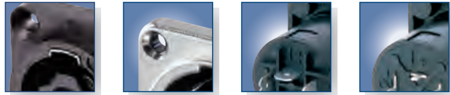
加固锁定区域 镍外壳 3/16"平插片 垂直PCB安装
